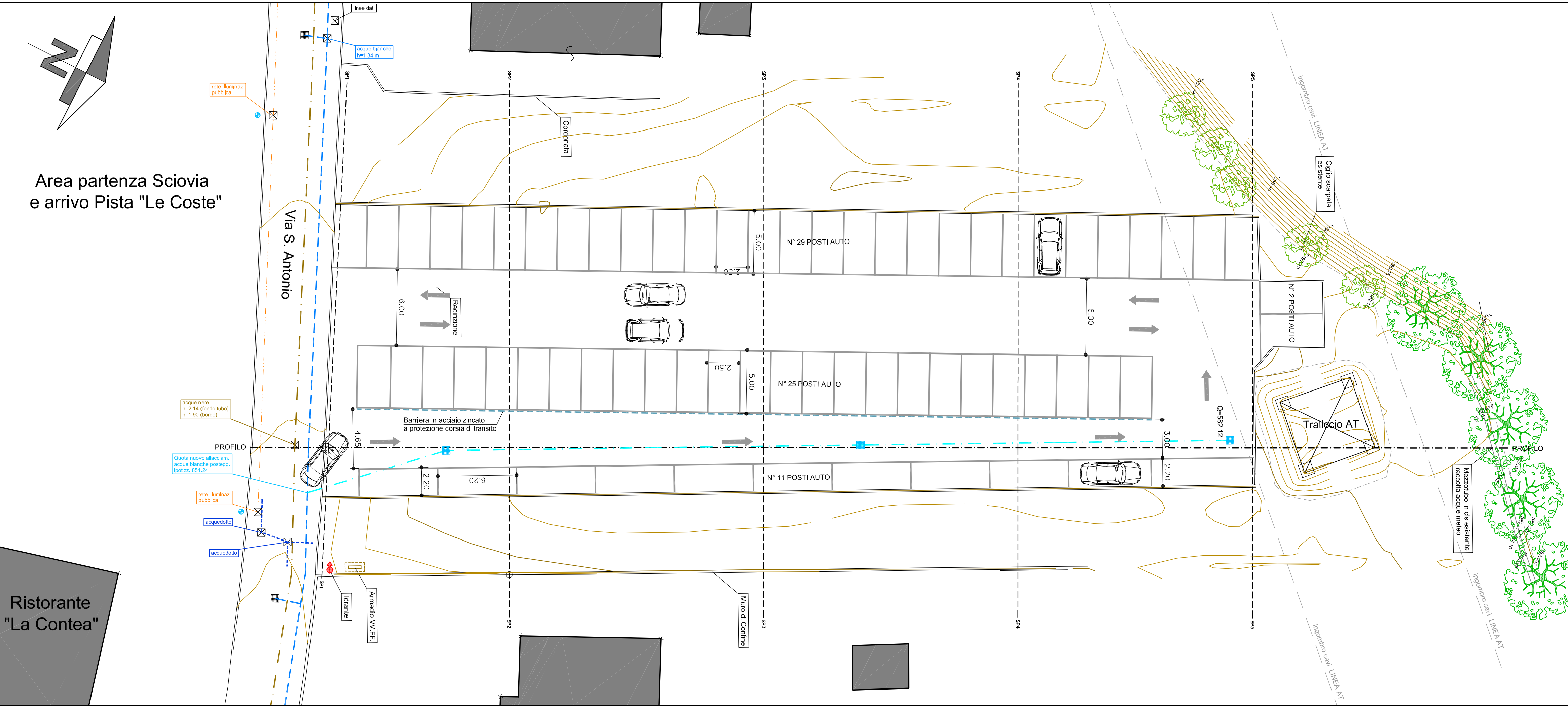
PLANIMETRIA di PROGETTO 1:200.-
